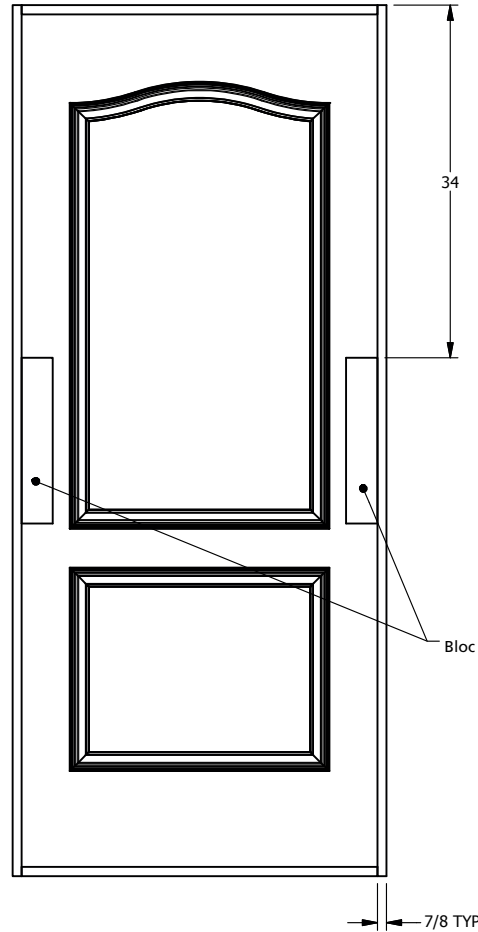
Position du bloc de poignée Dessin / vue intérieure de la porte
