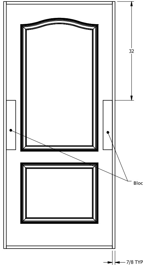
Position du bloc de poignée Dessin / vue intérieure de la porte
