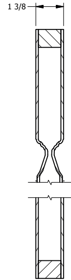
SECTION A-A
