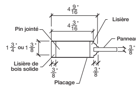
BATTANT PANNEAU PLAT
