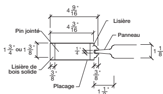
BATTANT PANNEAU SOLIDE PROFILÉ
