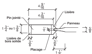
BATTANT PANNEAU PROFILÉ
